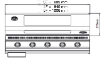
DIMENSIONI GENERALI
