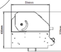
DIMENSIONI GENERALI
